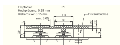
THT terminal inward
