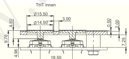
THT innen
