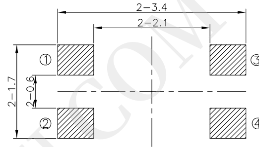
RECOMMENDED P.C.B. LAYOUT 安装尺寸图
