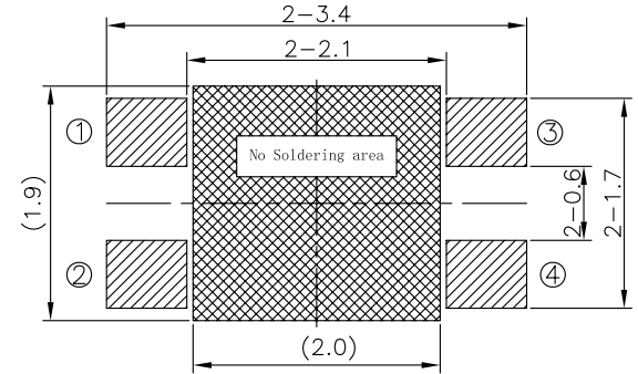
LAND PATTERN PLAN 印刷电路板焊盘参考图
