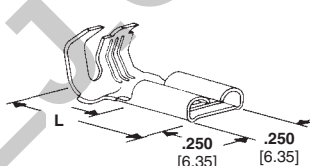
E — Premier Line, Tab-Lok Flag
