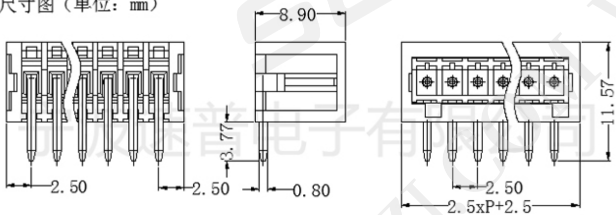
尺寸图 (单位: mm)
