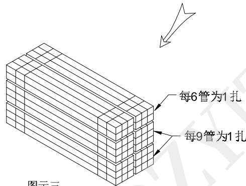
图示三 3.将每扎管子包扎
