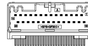
2*14PIN
