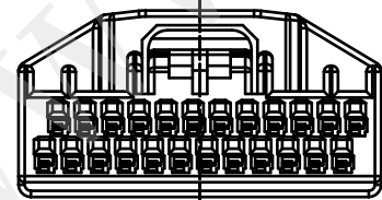
2*12PIN
