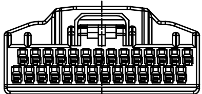
2*14PIN
