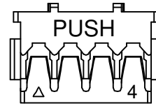
4Pin
