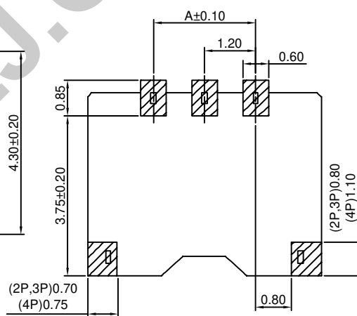
P.C.B LAYOUT
