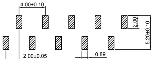
P.C.B LAYOUT
