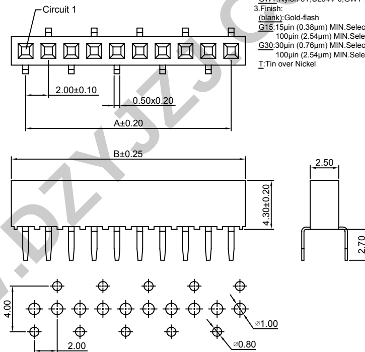
P.C.B LAYOUT
