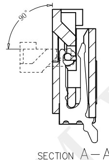
SECTION A-A
