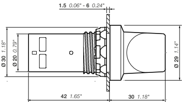
C3SS, 短手柄操作 尺寸 (mm, 英寸)
