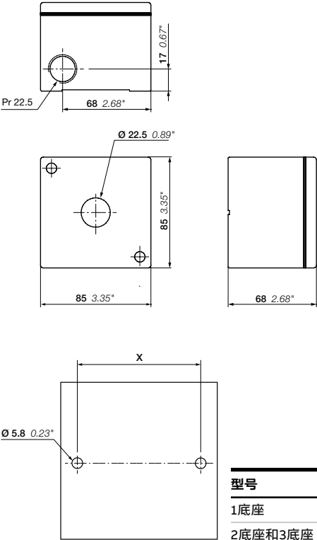
1、2、3底座KEM钻孔图
