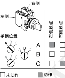
触点状态
