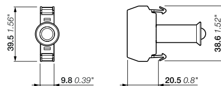
P9PL 尺寸 (mm, 英寸)
