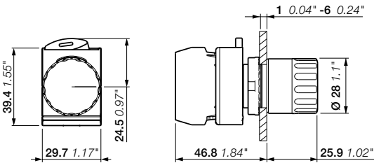
P9MPS 尺寸 (mm, 英寸)
