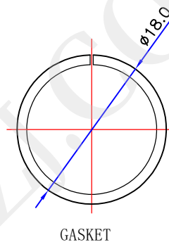
GASKET
