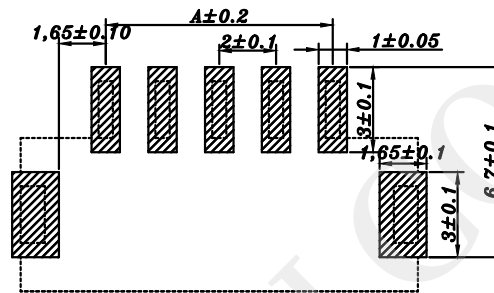
印制线路板
