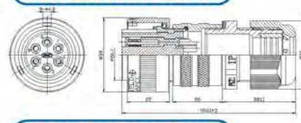
PLT3106A 20-15SC
