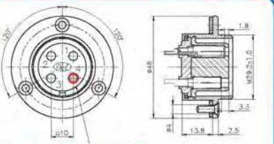
PLT-30-RF-R
