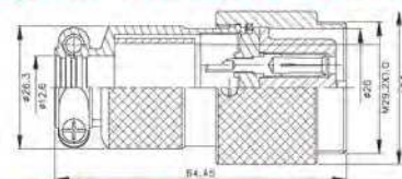
PLT-30-ADF-R
