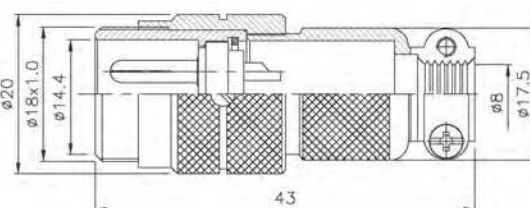
PLK-16-AD-R
