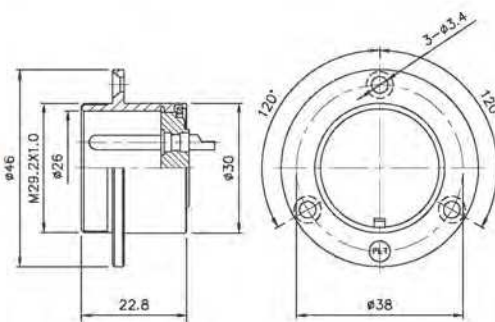
PLT-30-R-R
