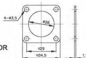
PAT A-589PX
