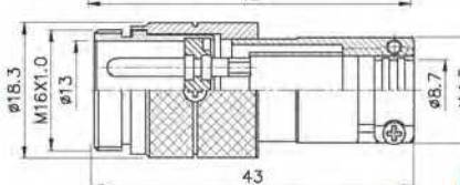
PLT-16◆-ADA-R
