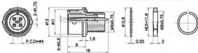
WPM-94-RF-R
