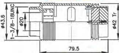
PLS-42◆-PF1
