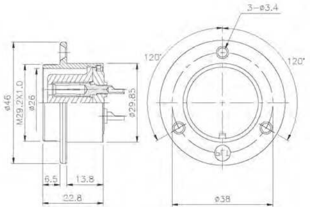
PLK-30-RF-R
