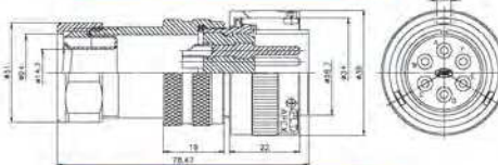
PLT3106A 20-15PG4
