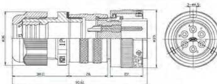
PLT3106A 20-15PC
