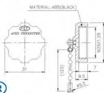
PLT-25◆-WGPM3-R
