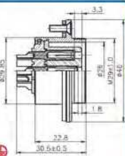
PLT-307E-RF-R
