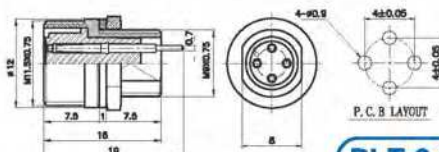
PLT-9-RPCB
