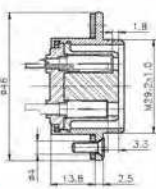
PLT-304E-RF-R
