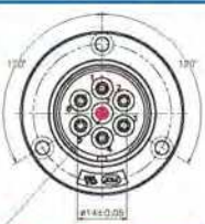
PLT-304E-RF-R
