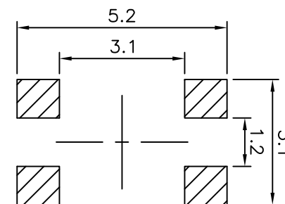
PCB. 焊接图
