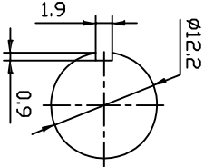
安装尺寸 (Mounting)
