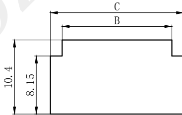
安装尺寸图
